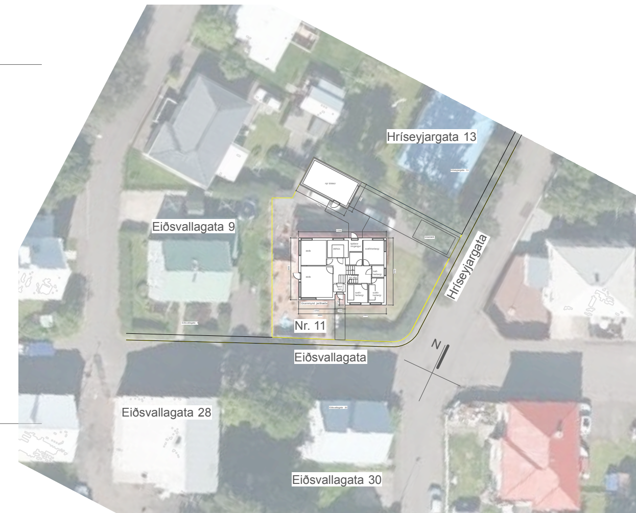
8 AFSTÖÐUMYND Scale: 1:500
