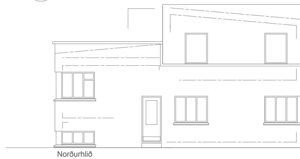
5 ÚTLIT NORÐURHLIÐAR Scale: 1:100
