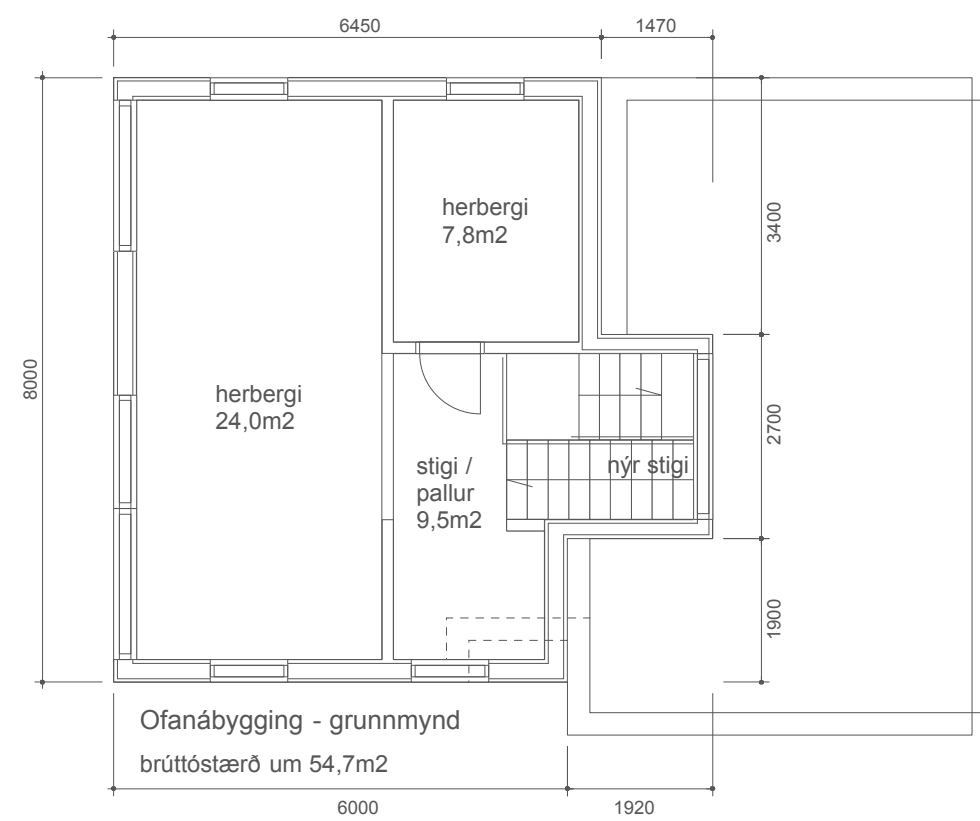
3 GRUNNMYND NÝRRAR OFANÁBYGGINGAR Scale: 1:100
